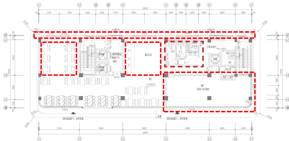
二层平面图 1:100
