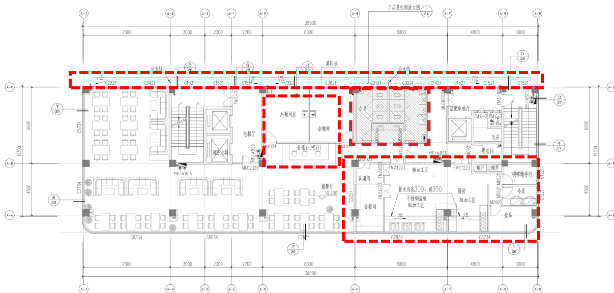
三层平面图 1:100
