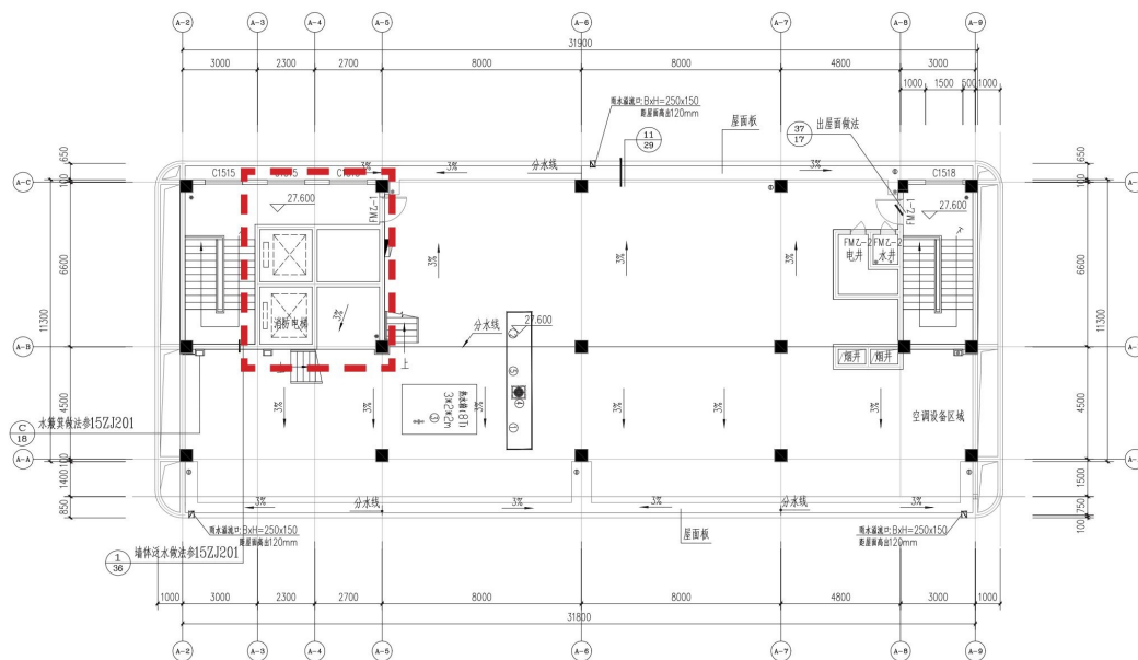
屋顶平面图 1:100
