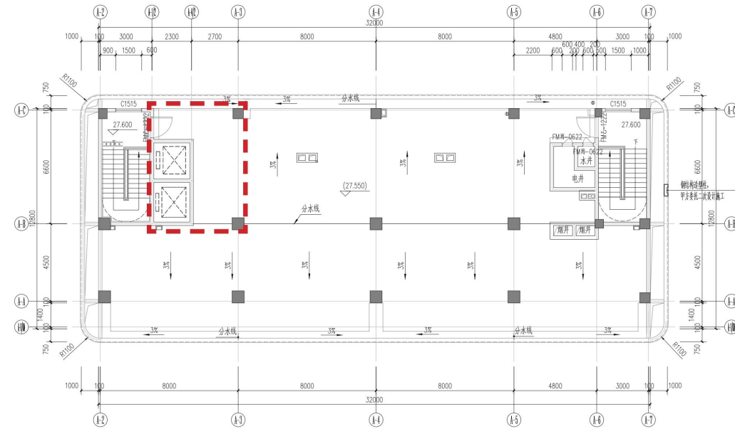
屋顶平面图 1:100
