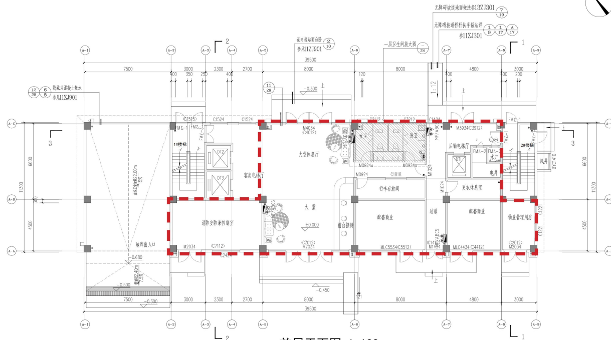
首层平面图 1:100
