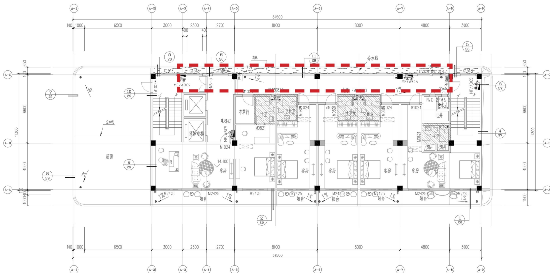
四层平面图 1:100
