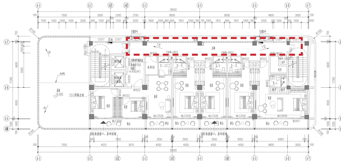
四层平面图 1:100
