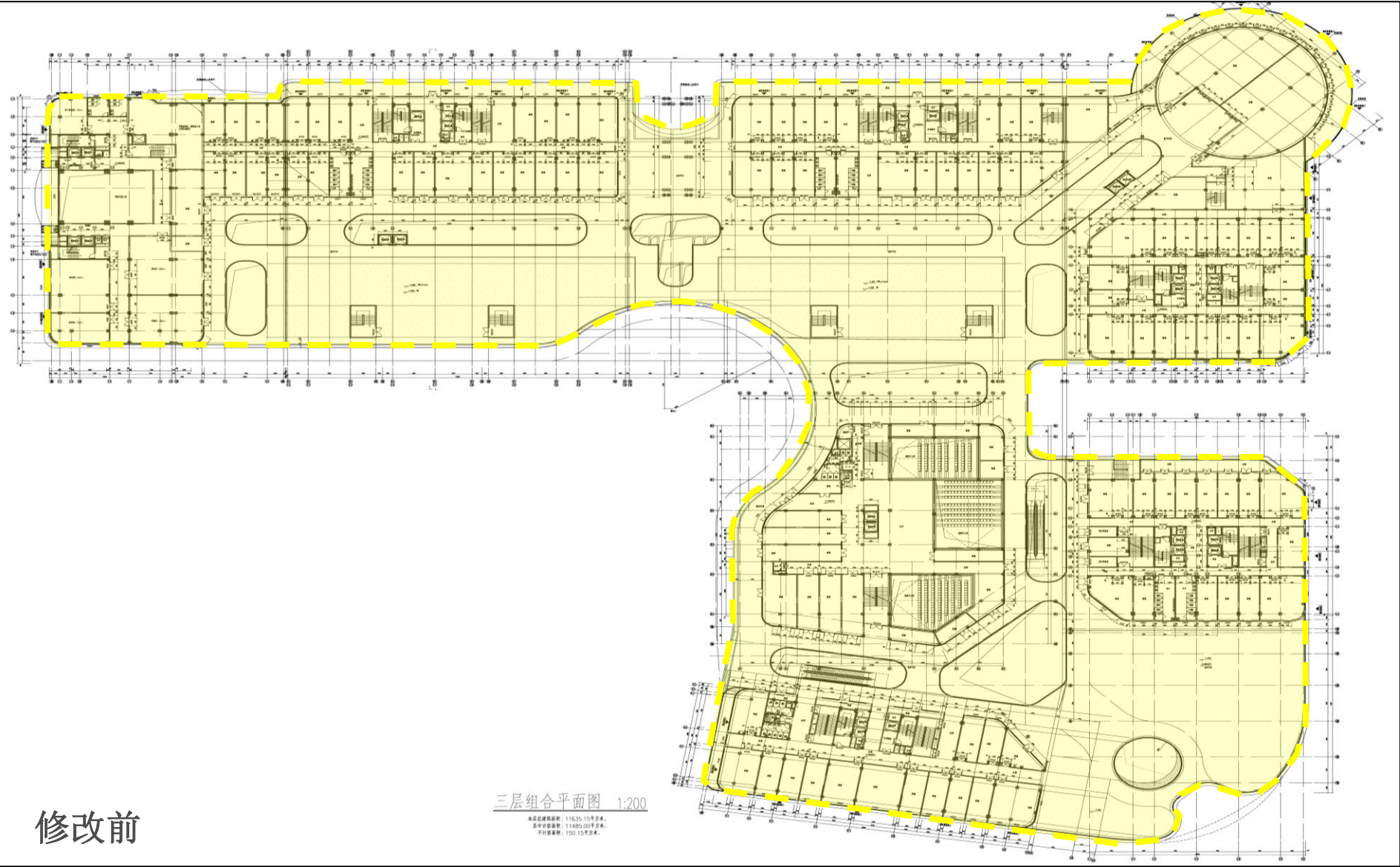
三层平面图
