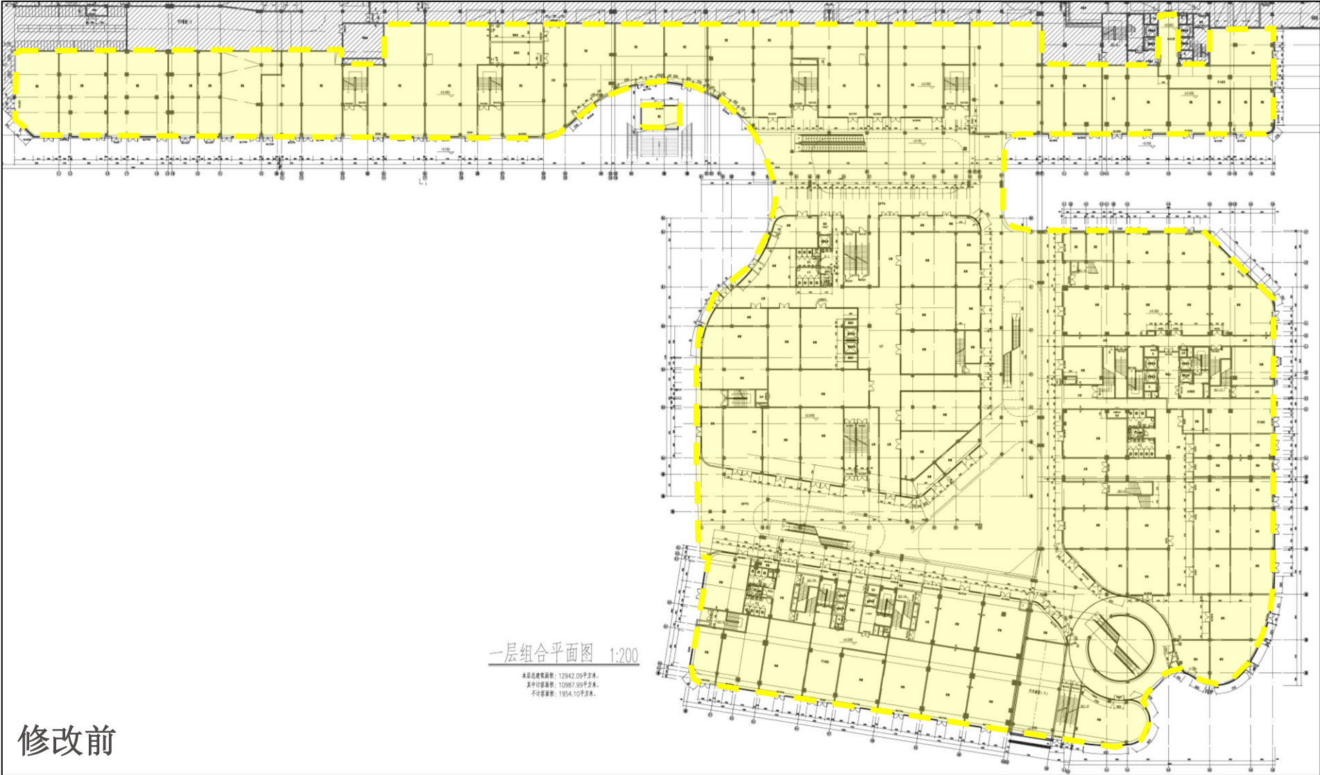
一层平面图
