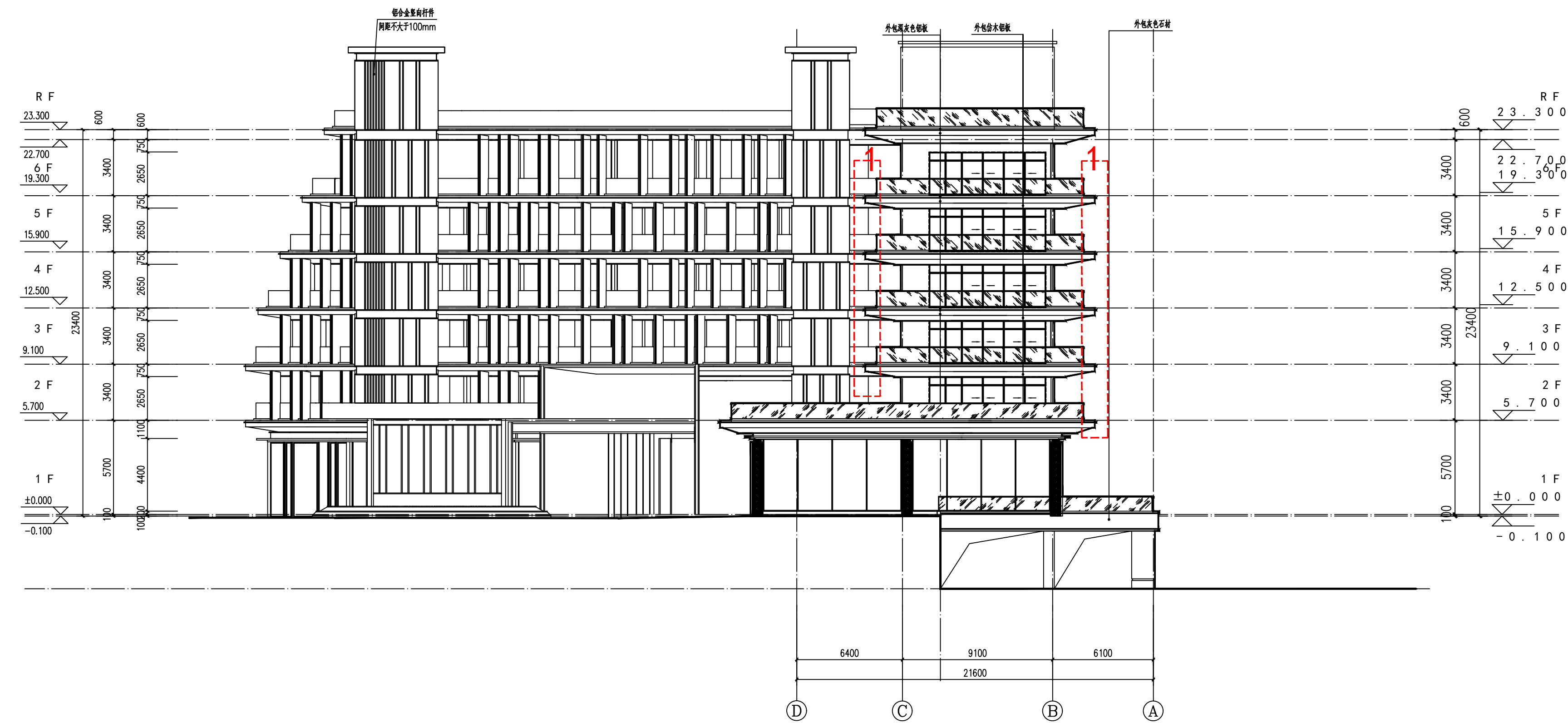
①~④轴立面图
