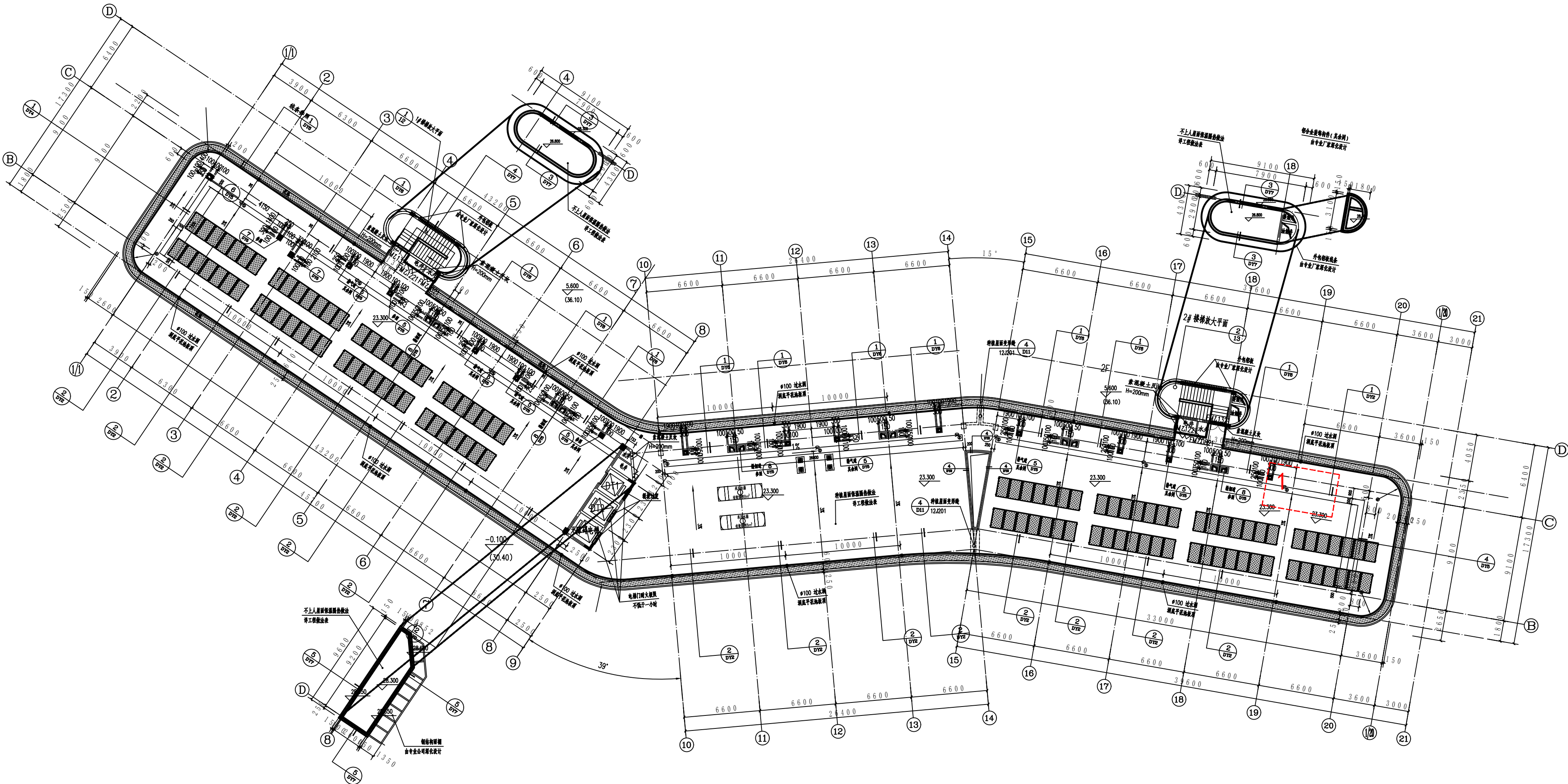
屋顶层平面图 屋顶层面积: 74.12m²
