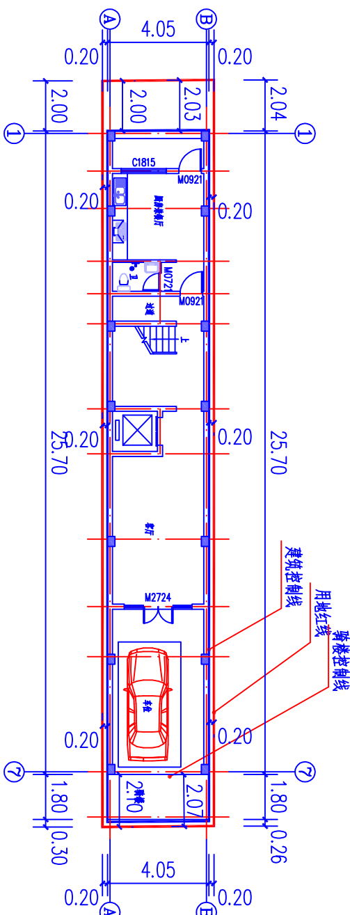
变更前首层总平面图 1:200
