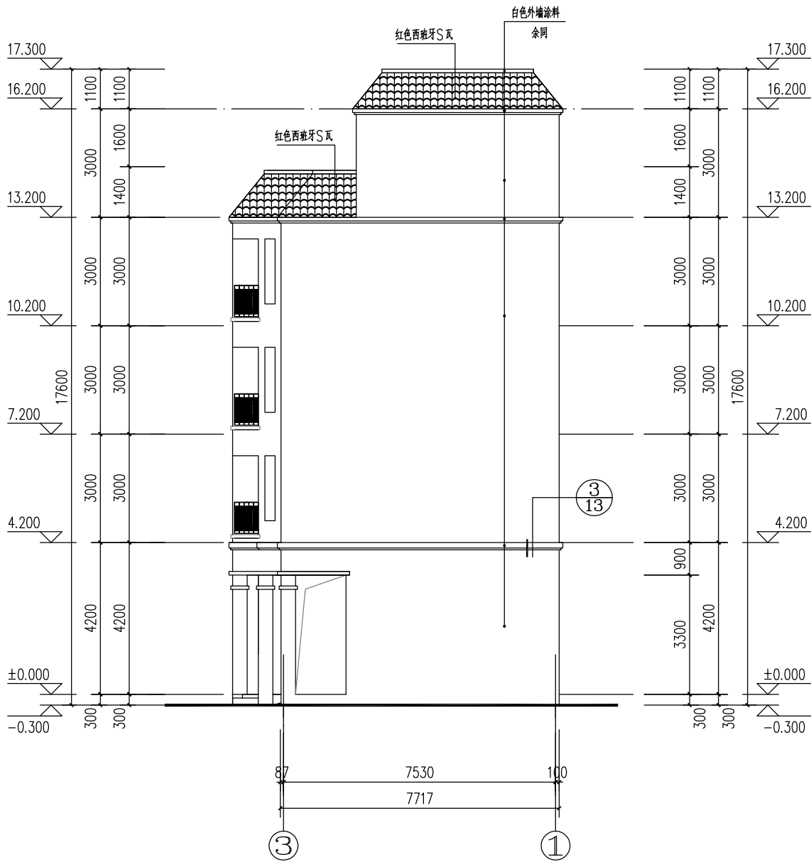
③~①轴立面图 1:100
