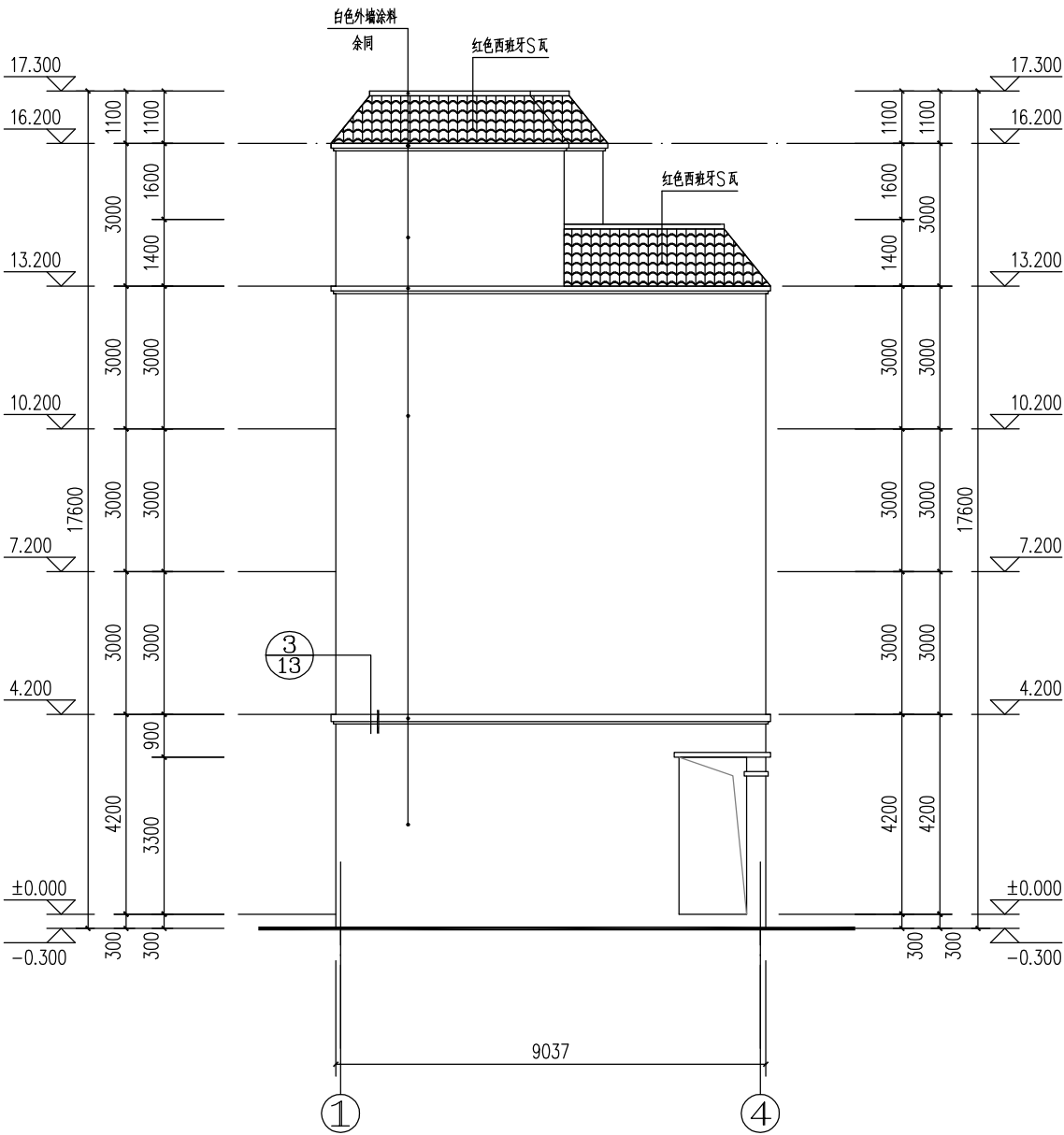
①~④轴立面图 1:100
