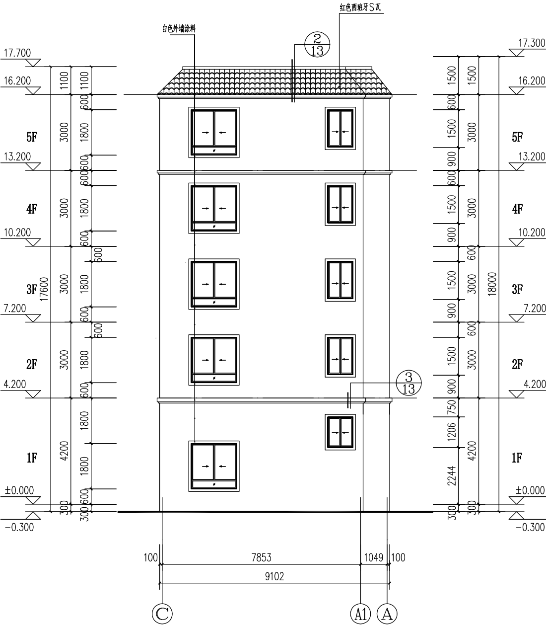
④～⑥轴立面图 1:100
