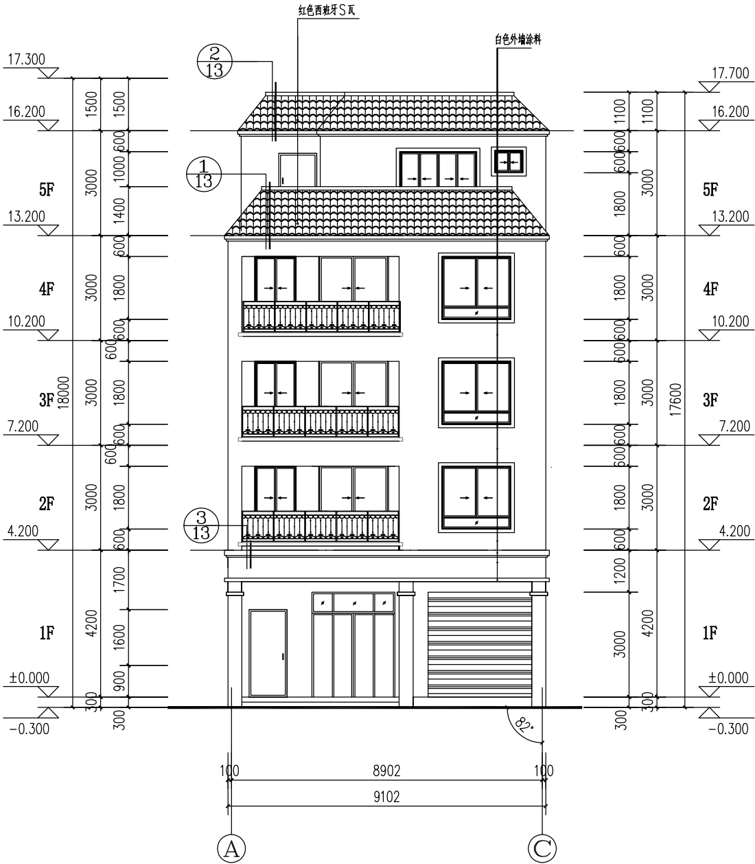
①～③轴立面图 1:100
