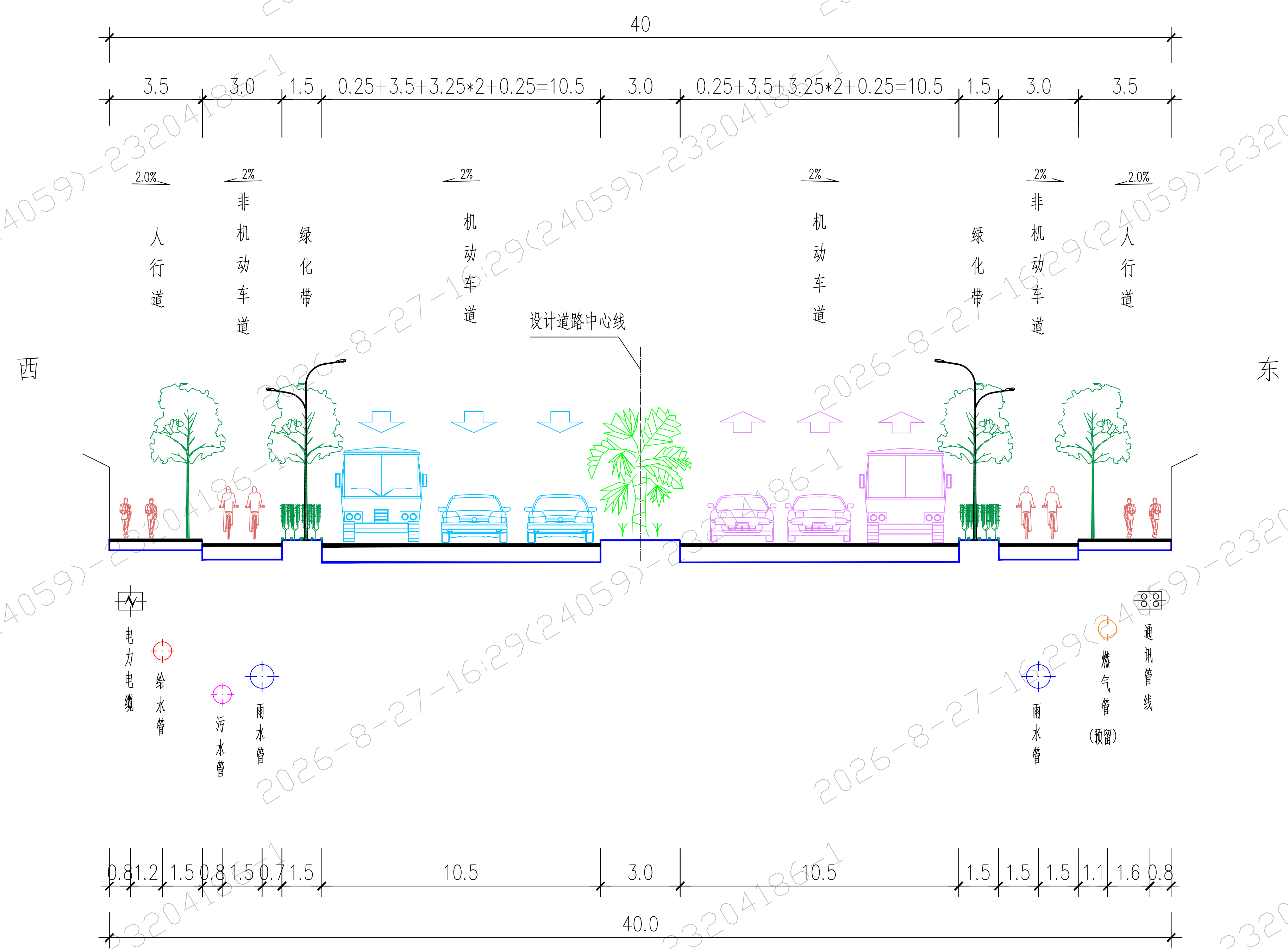
管线综合横断面图 海声路
