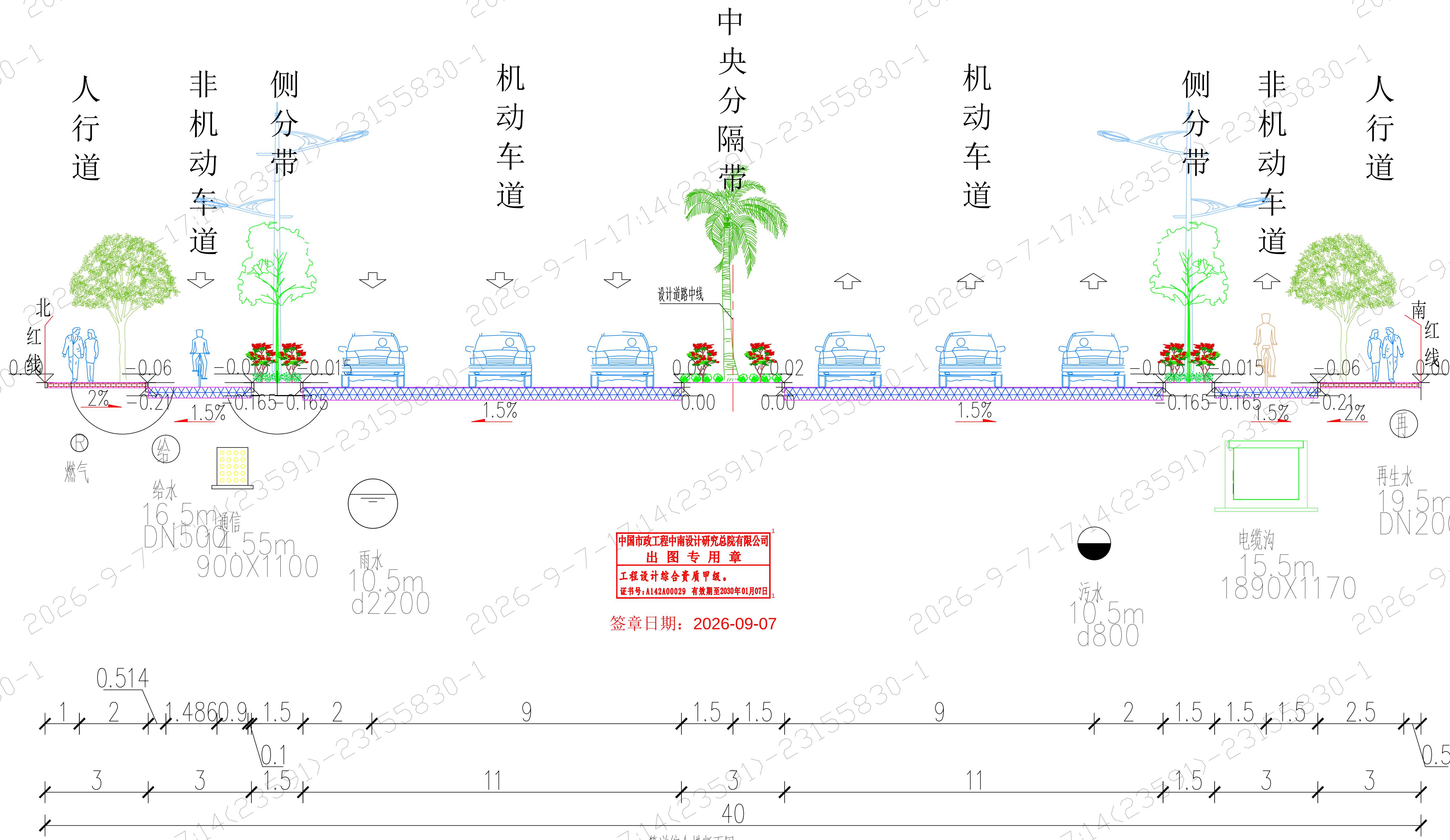
管道综合横断面图
