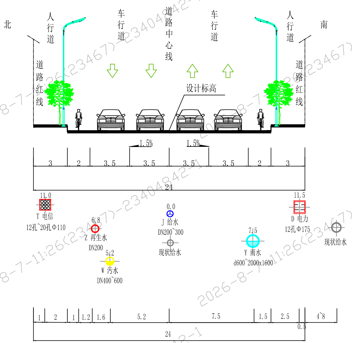
森海路管线综合横断面图
