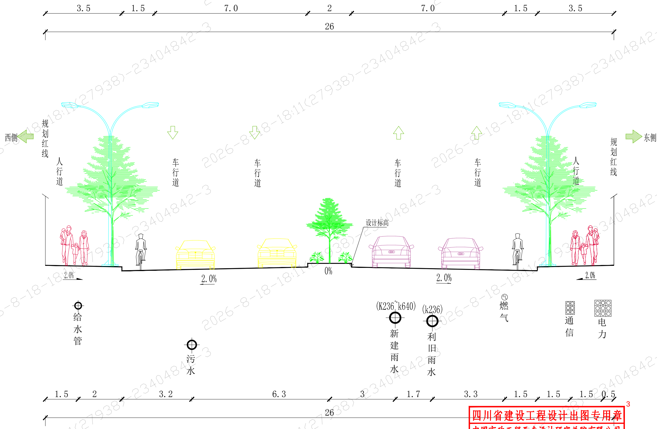
道路标准横断面图（红线26m）
