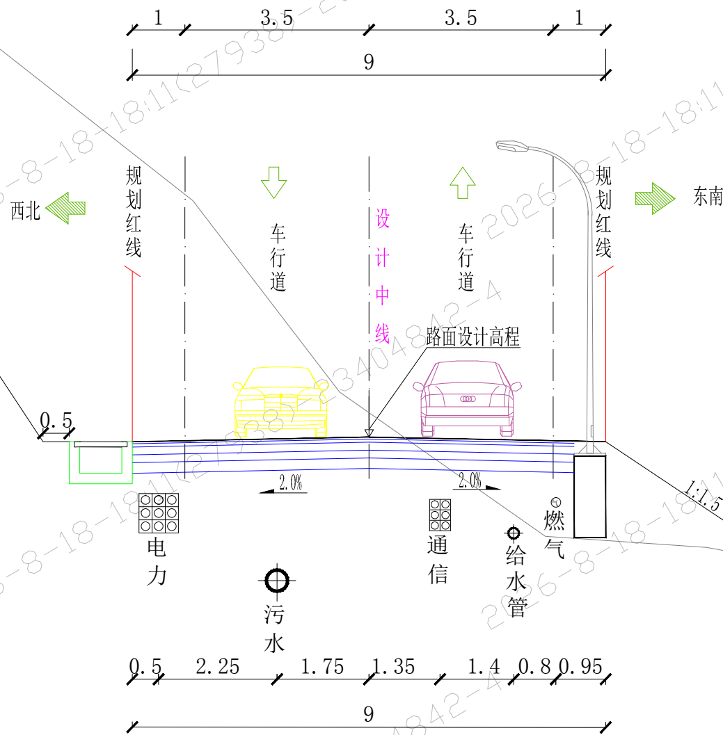
管道综合横断面图 (红线9m)
