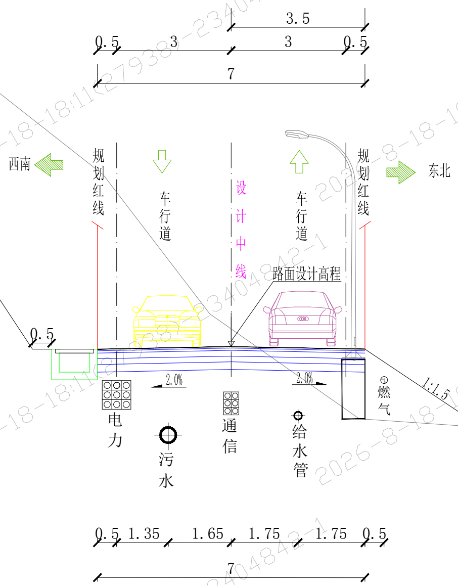
管道综合横断面图（红线7m）
