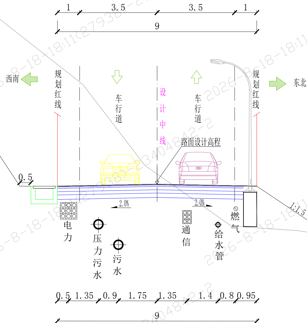
管道综合横断面图（红线9m）
