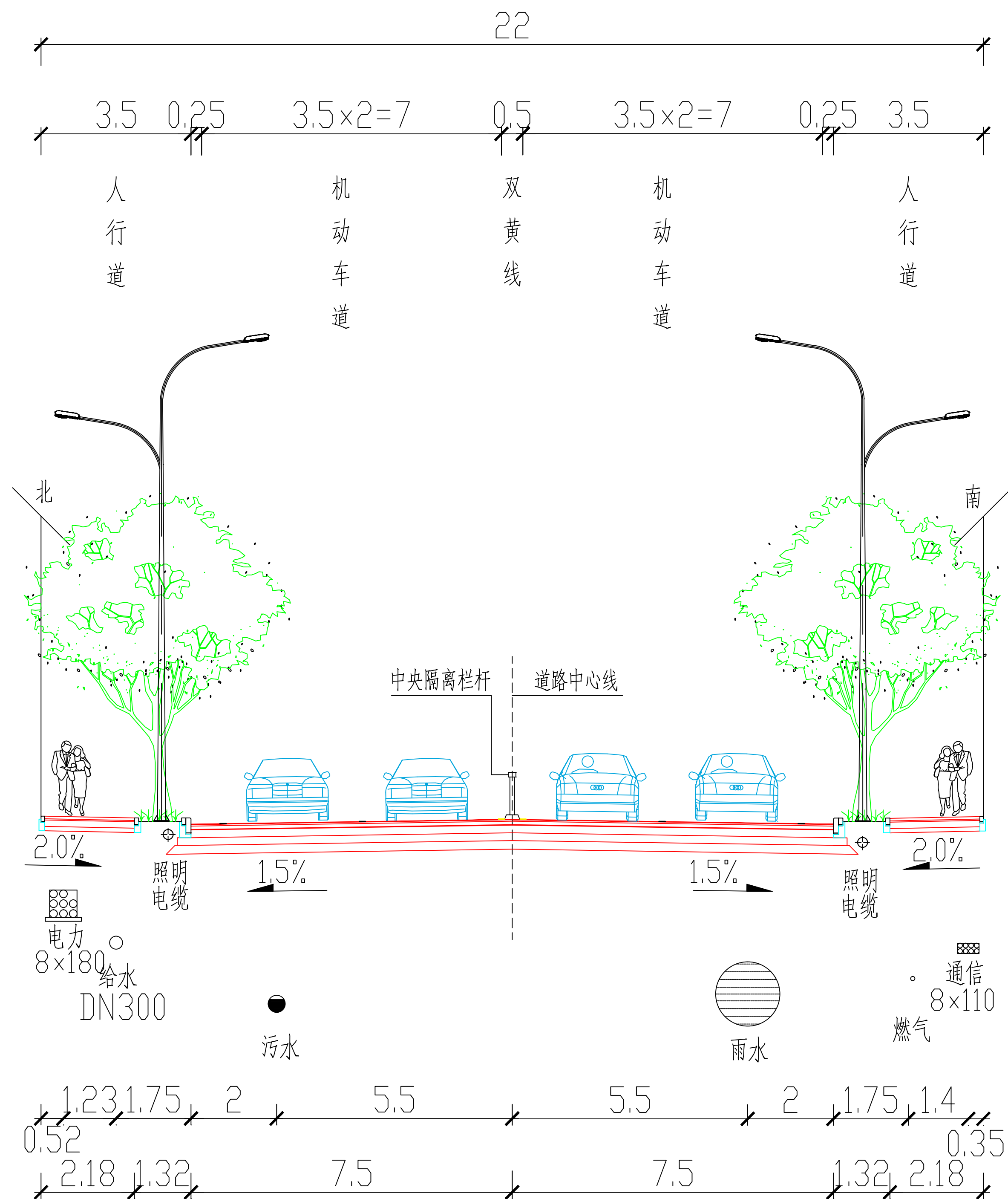
22米综合管位标准横断面图 (适用于临春路北段22米道路标准横断面)
