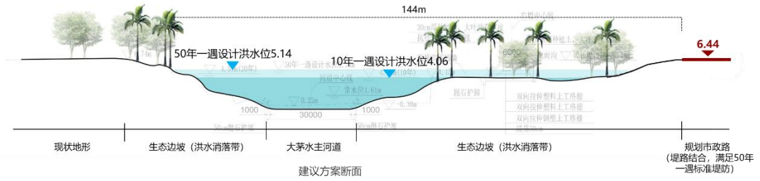
图 3-4 堤路结合规划断面图
