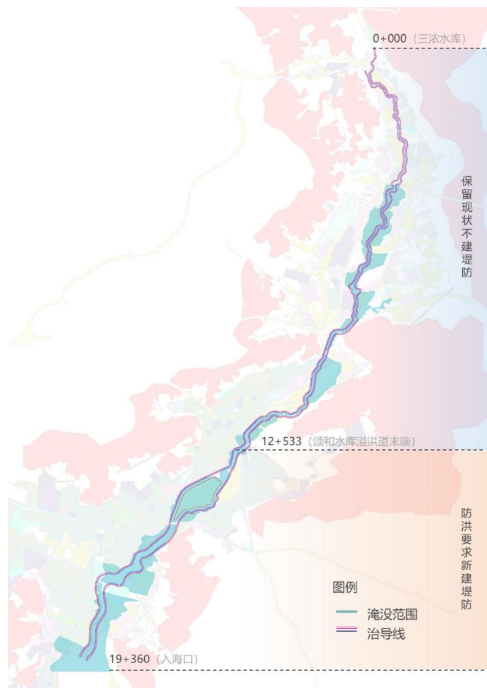
图 3-3 河道岸线规划总体情况
