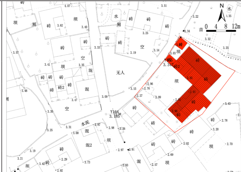
总平面图
