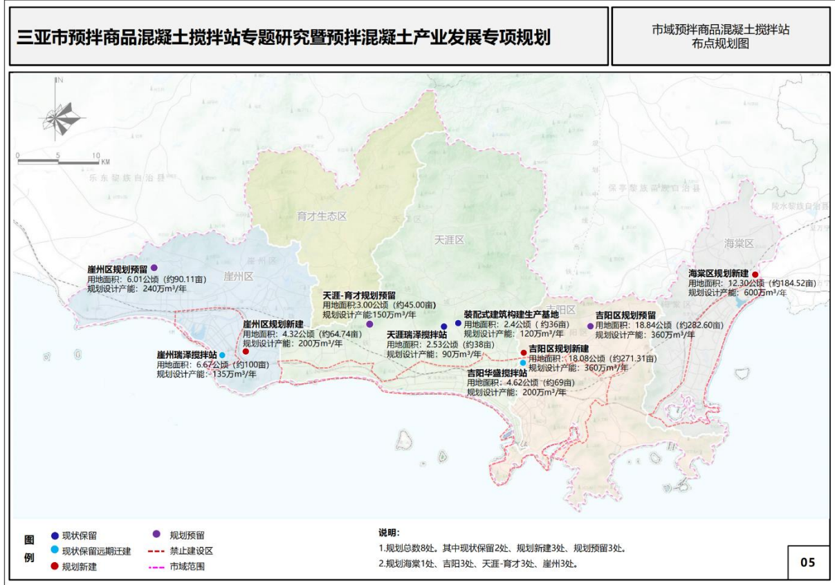
图 3-1 三亚市混凝土搅拌站规划分布图
