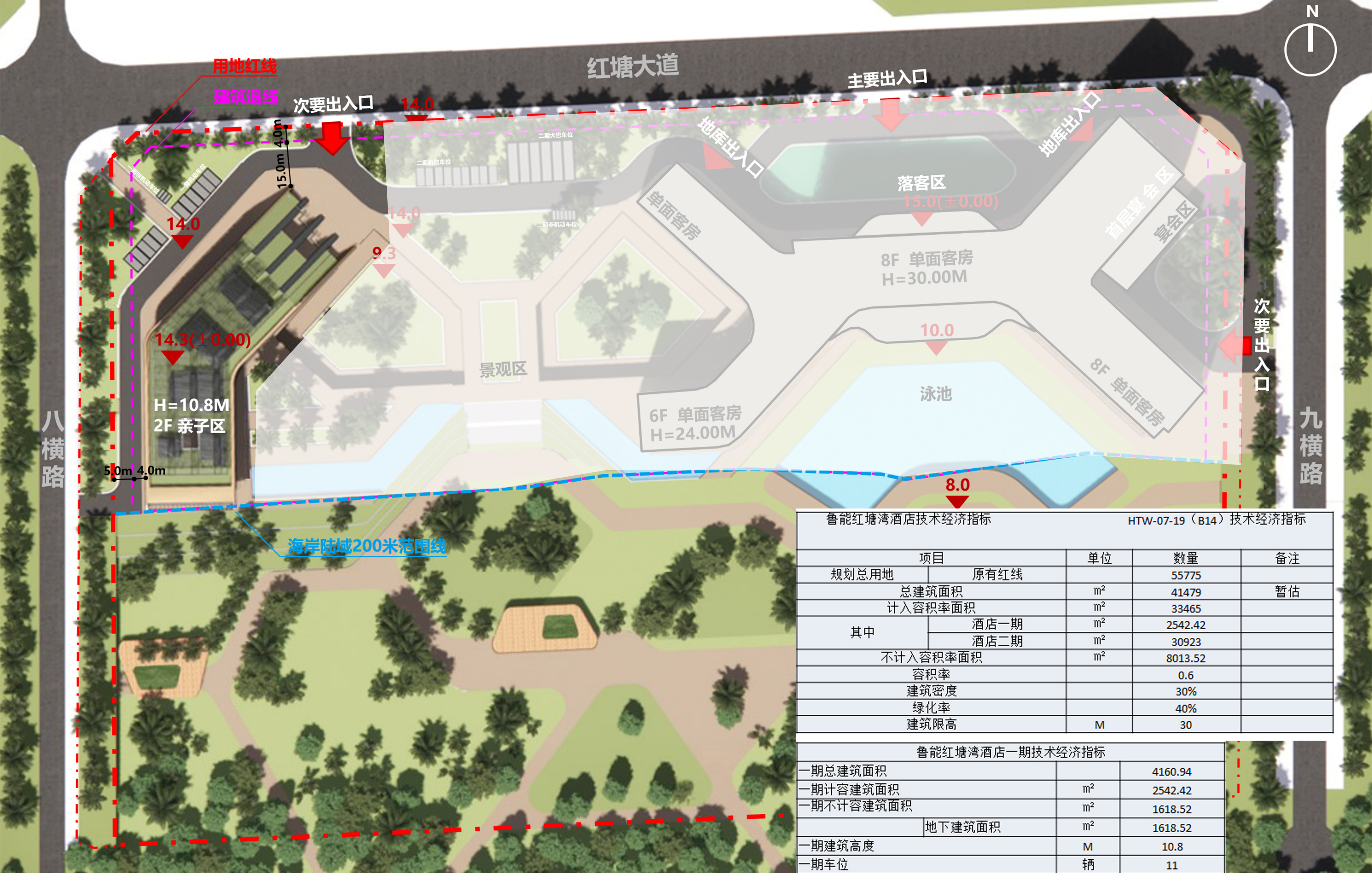
MASTERPLAN | 总平面
